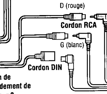
Cordon prolongateur (fourni avec le CX-DP880U)
